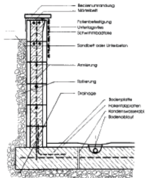
Symbolzeichnung
